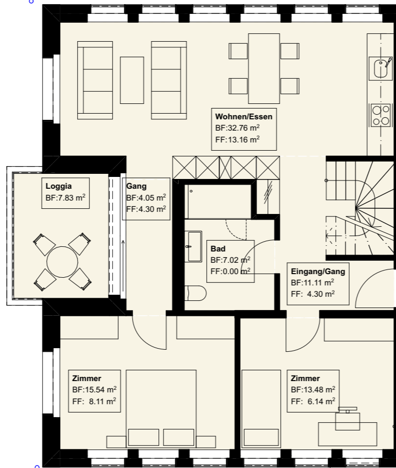
2. OBERGESCHOSS
